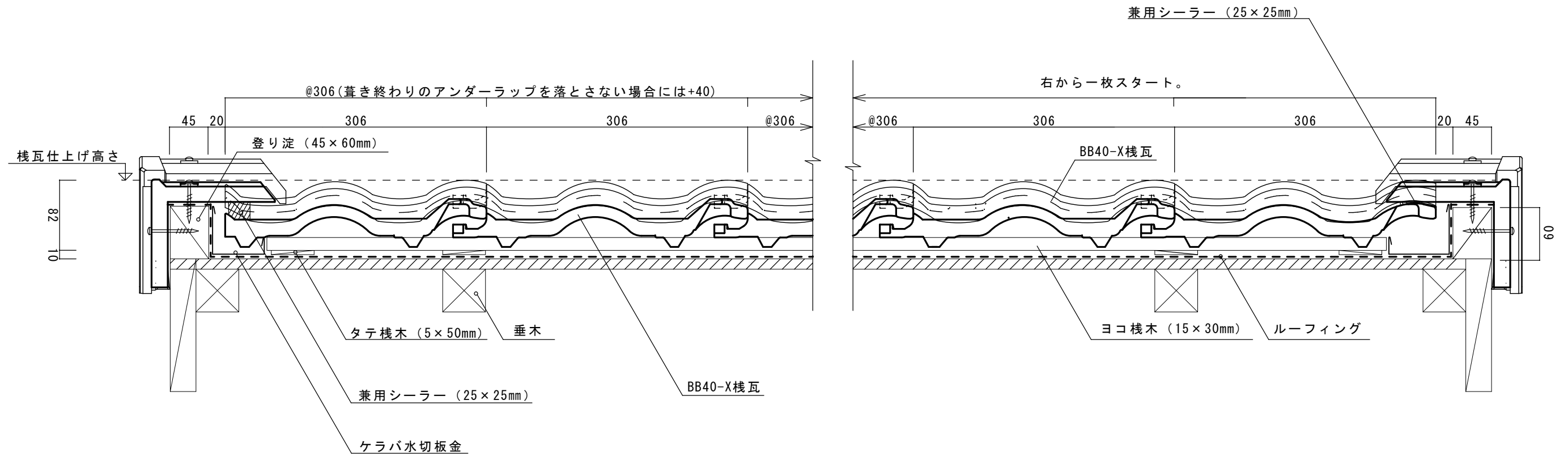
袖部横断面 縮尺 1 : 5
