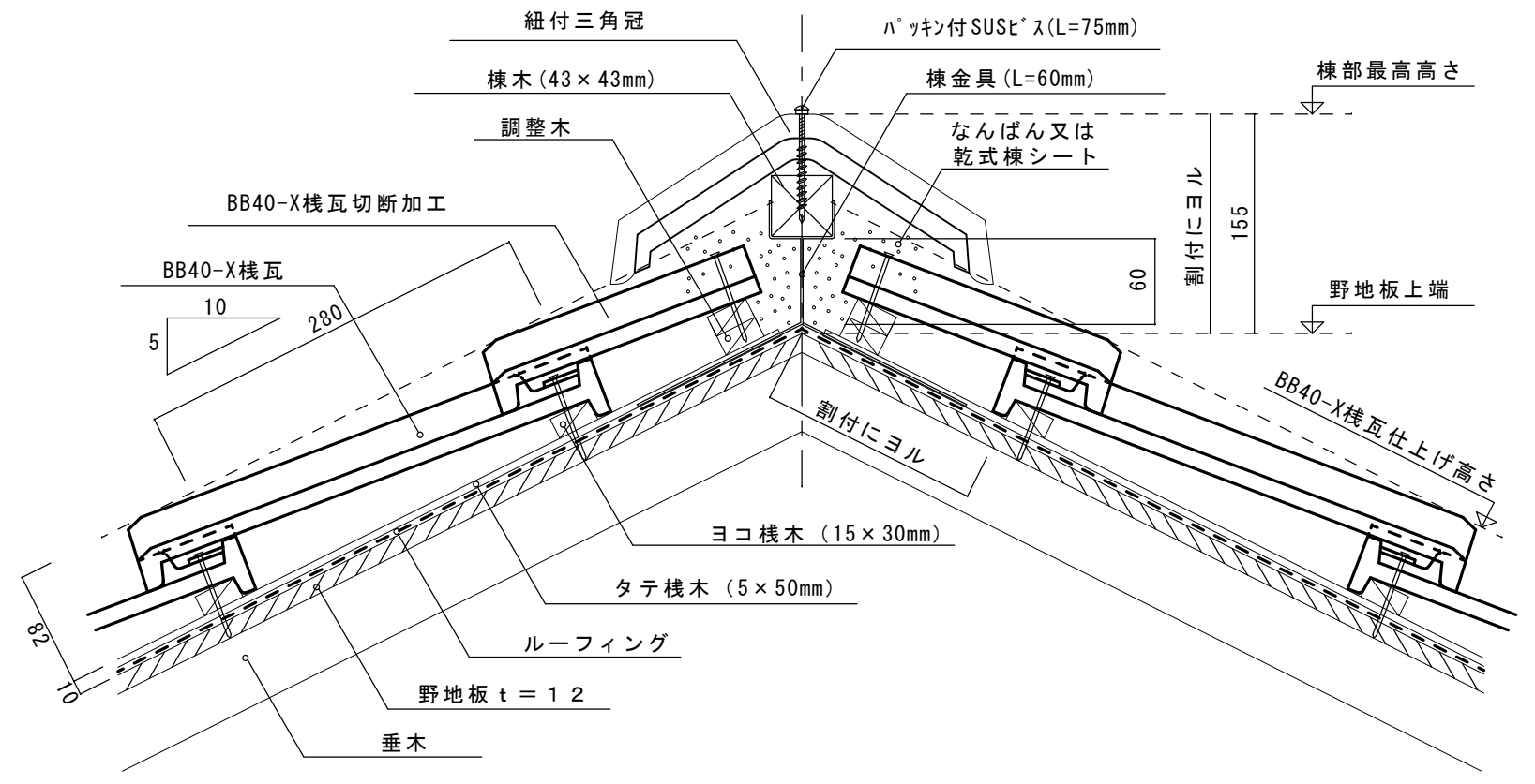
大棟部 縮尺 1 : 5
