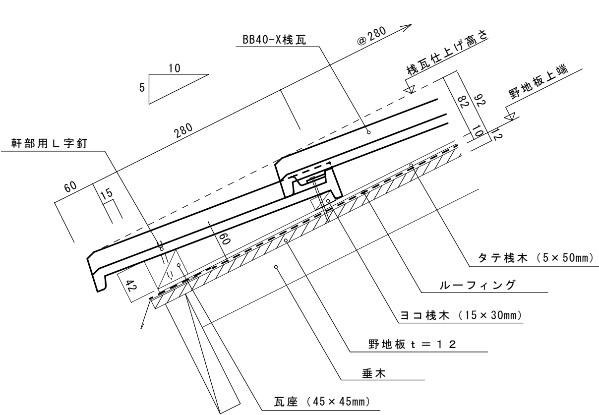
袖部横断面 縮尺 1 : 5
